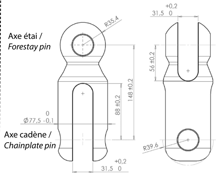
Pour modèles C480, C520, C530 montés sur cadène en aluminium For C480, C520, C530 models fitted on an aluminium chainplate
