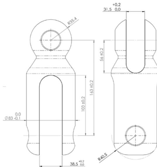
Pour modèles C480, C520, C530 montés sur cadène en aluminium For C480, C520, C530 models fitted on an aluminium chainplate
